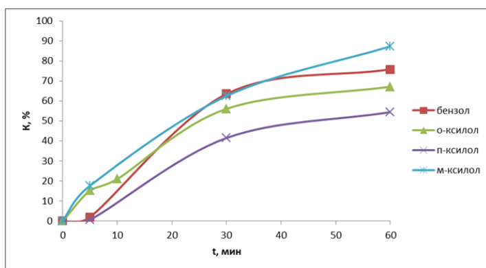
Рис.1. Зависимость конверсии от времени гидрирования для изомерных ксилолов (3 атм и 170°C) на катализаторе La-Ag/МС.
