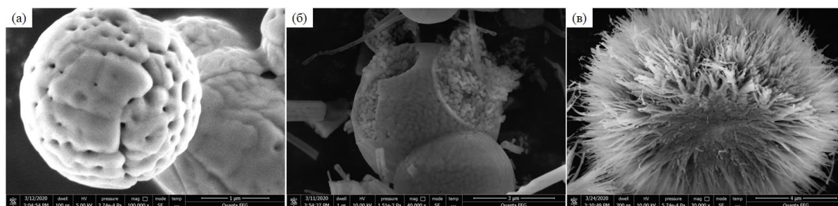
Рисунок – РЭМ фотографии образцов \alpha - \text{Al}_2\text{O}_3 , T_{\text{ГТС}} = 90 (а), 110 (б) и 130 °С (в)
