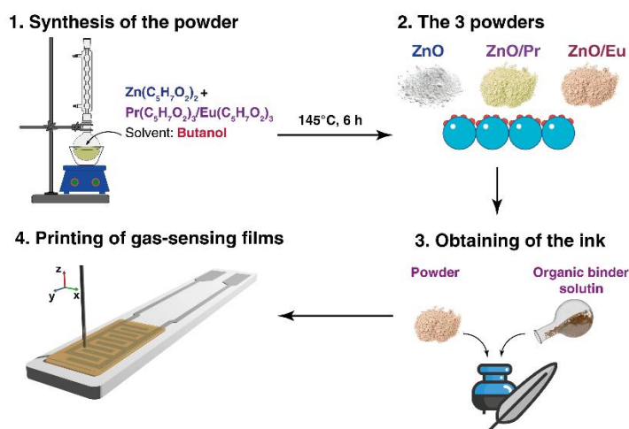
Рис. 1. Схема синтеза газочувствительных материалов на основе ZnO и нанесения покрытий на специальные датчики
