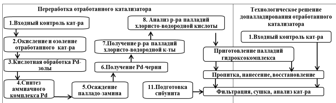
Рисунок 2 – Варианты переработки отработанного катализатора
