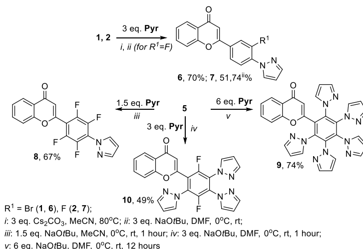
Схема 2. Трансформации фторсодержащих флавонов с пиразолом
