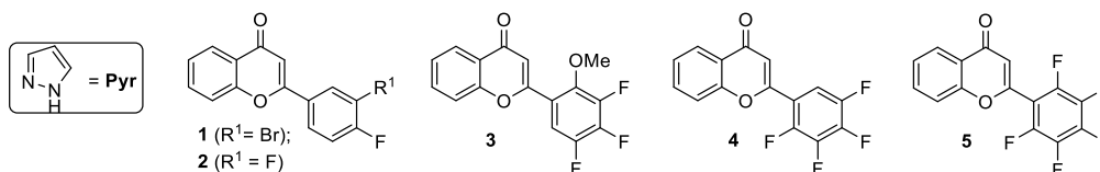
Схема 1. Структуры фторарилсодержащих хромонов 1-5
