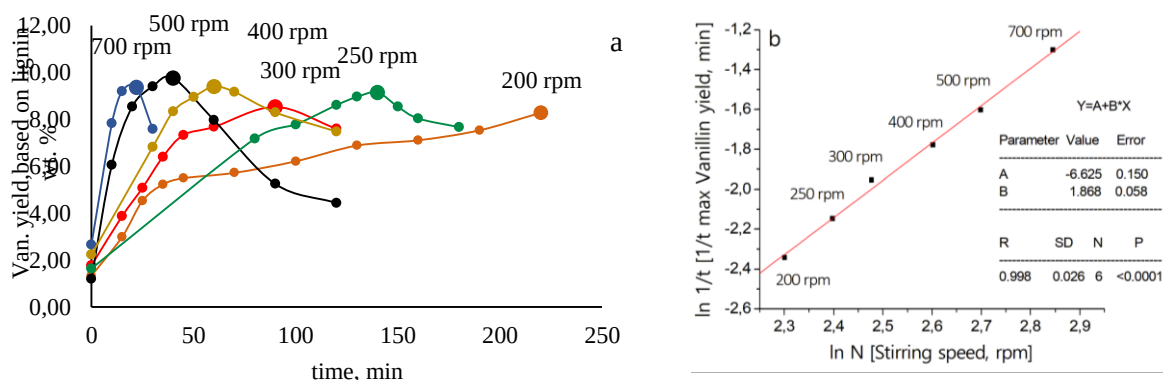
Рис. 1. Влияние скорости перемешивания на динамику накопления ванилина (a); логарифмическая зависимость скорости накопления ванилина (оценена как 1/t_{\max} , обратное время достижения максимальной концентрации ванилина) от скорости вращения мешалки (b).
