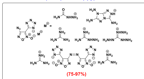
Соли (тетразолил)фуроксанов
