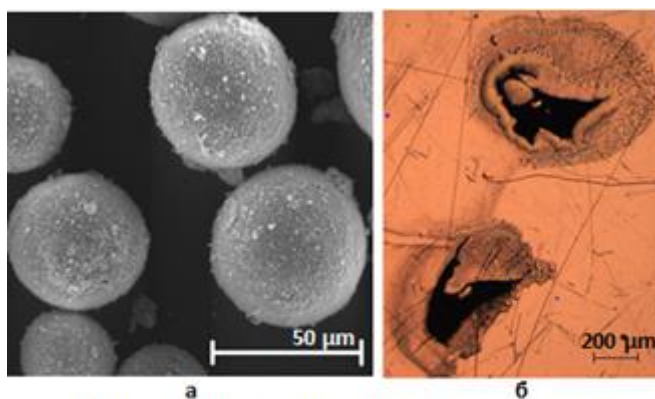
Рисунок - Керамический порошок (а) и микроструктура лазерной наплавки (б)
