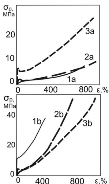
Рис.1 Зависимость напряжения от относительной деформации для образцов на базе ПЭ-1000 (1а, 1б), ПЭ-2000(2а, 2б) и ПЭ-3500 (3а, 3б), отвержденных ПЭ (а) и МОСА (б).
