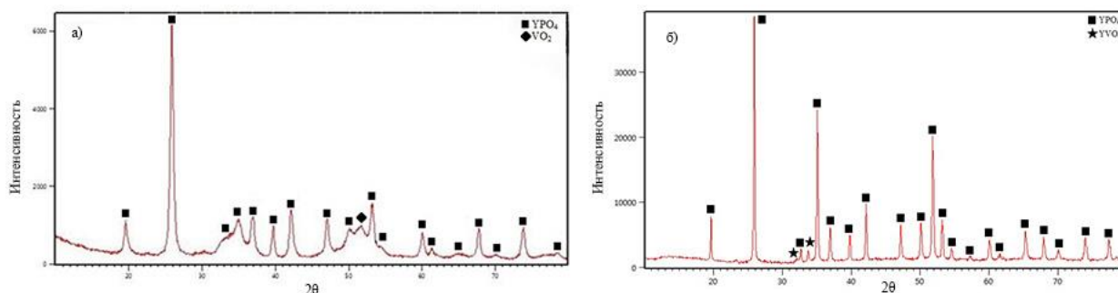
Рис. 1. Рентгеновские дифрактограммы \text{YV}_{0,1}\text{P}_{0,9}\text{O}_4 : микроволновый синтез (а), спрей-пиролиз (б)
