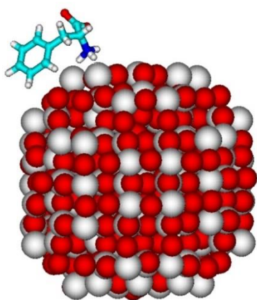
Рис. 1. Строение комплекса «Phe - \text{TiO}_2 »
