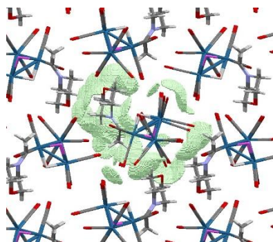
Рис. 1 Комплементарное поле кластера
