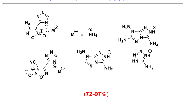
Соли (1,2,4-триазолил)фуроксанов
