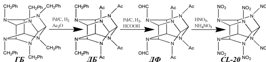
Рисунок 1 – Схема синтеза CL-20
